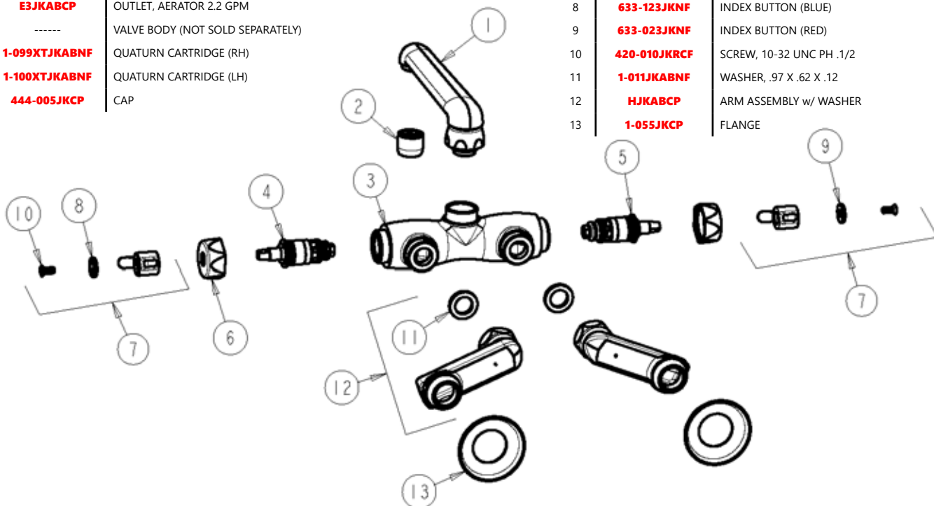
ACTUATOR ASSEMBLY 665-190JKABNF
